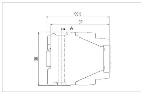
Standard DIN housing format
