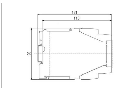
Long DIN housing format
